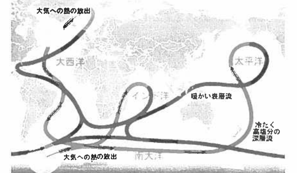
図2 深層大循環の模式図
