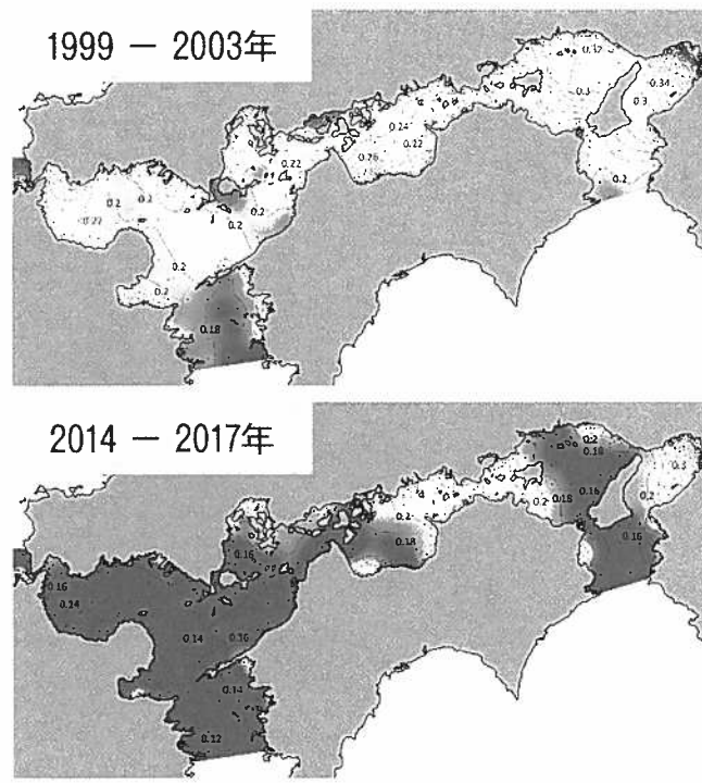
図4 全窒素濃度(表層)水平分布. グレーの海域は0.2mg/L以下. 藤原より
