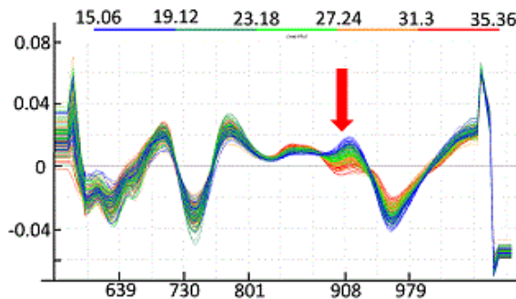
図6 養殖マサバの吸光度2次微分近赤外スペクトル(総脂質を5段階に色分け)
