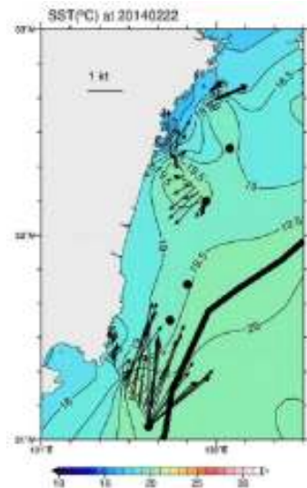
図2:水試日報の詳細図 (色は水温、矢印は潮流、太実線は黒潮流軸)
